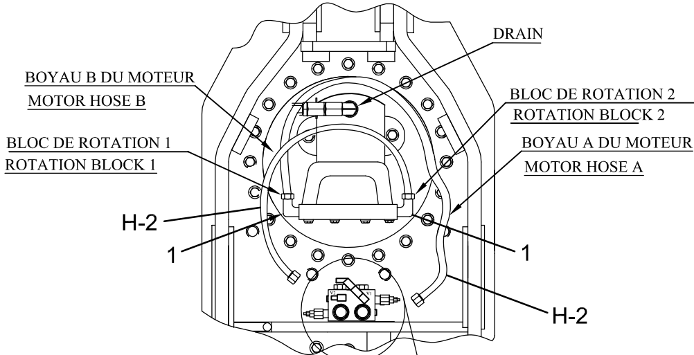
SCHEMA DU MOTEUR VUE FACE À L'ACCOUPLERMENT MOTOR DRAWING FRONT ATTACHMENT SIGHT
