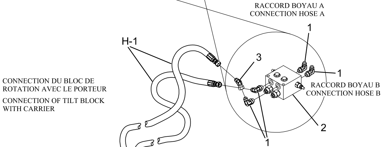
SCHEMA DU BLOC DE ROTATION TILT BLOCK DRAWING
