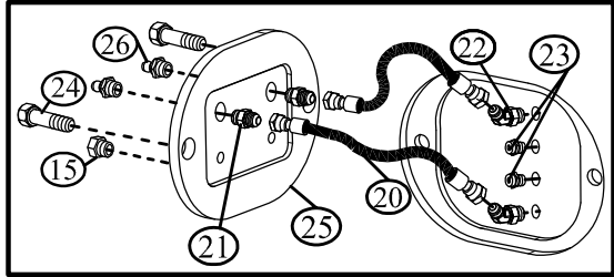
Panneau des boyaux à graisse / Grease hose panel
